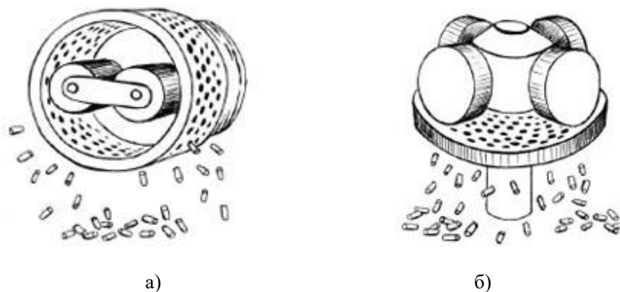
Рисунок 4 – Прес з круглою а) та плоскою б) матрицями для виготовлення пелет
