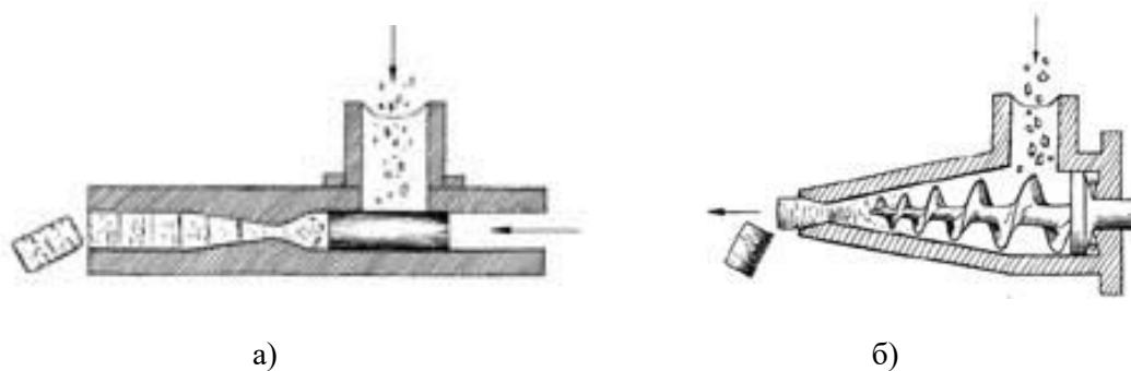
Рисунок 3 – Поршневий а) та шнековий б) прес для виготовлення брикетів
