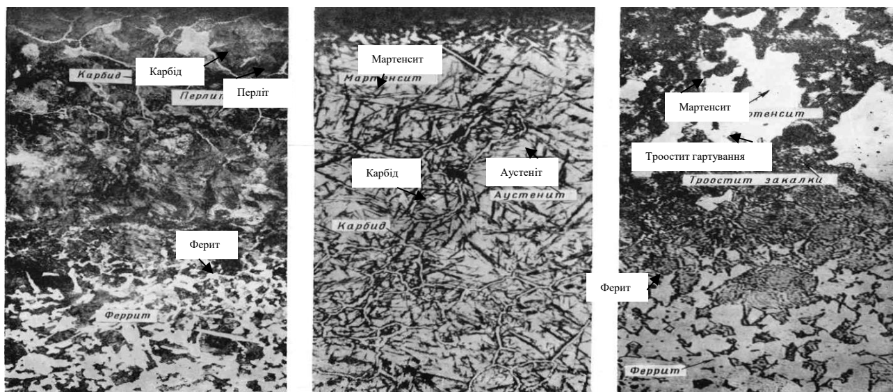
Рис. 1. Мікроструктури цементованої сталі
