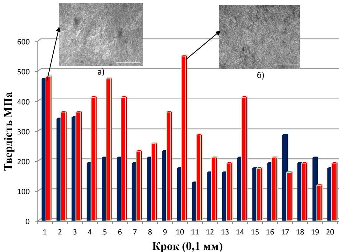
Рисунок 1 – Характер розподілу мікротвердості наплавленого шару: а) дрiт 30ХГСА; б) дрiт 30ХГСА з ферованадієм
