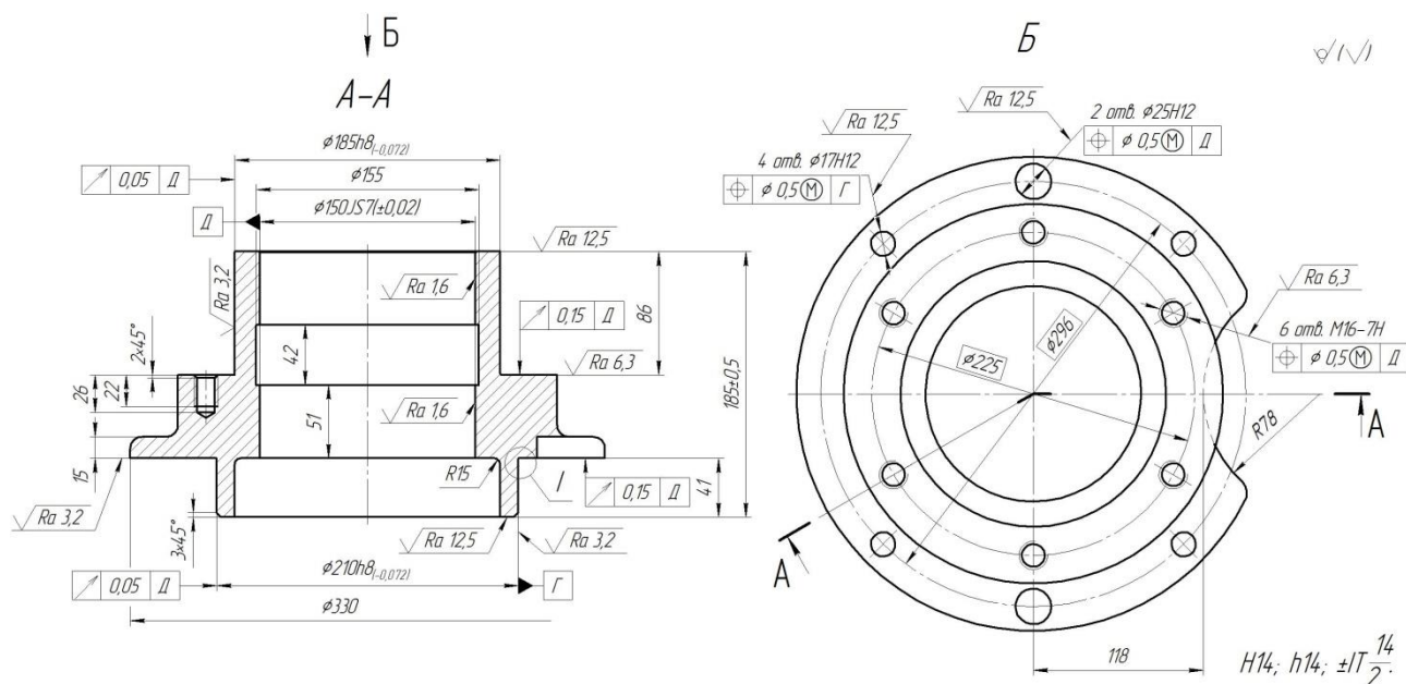
Рисунок 1 – Креслення деталі
