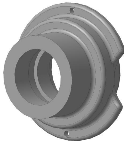
Рисунок 9 – 3D-модель заготовки, виготовленої литтям в піщано-глинисті форми з машинним формуванням суміші
